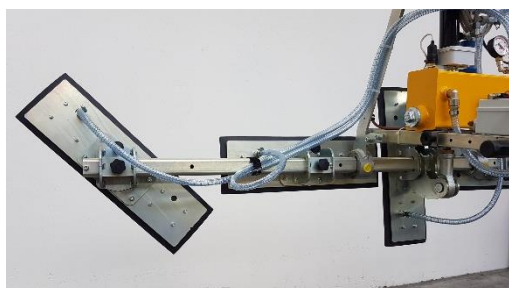
Supporto per rotazione rapida delle piastre
